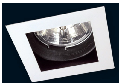
Cod:E4111 Embutido para Ar111 1Luz Anti deslumbrante Medidas:16x16x6,5cm Color:Blanco mate, interior negro
